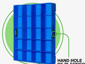
CHAROLA CHAROLA / PLÁSTICO CORRUGADO AZUL 5mm 720 MM X 540 MM MEDIDAS EXTERNAS: 36 CAVIDADES 930 mm 181 mm 770 mm 176 mm 126 mm HAND HOLE DE PLÁSTICO
