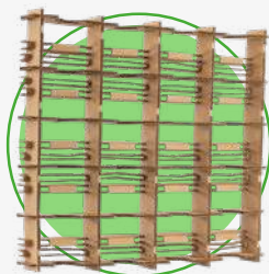
REJILLA CAVIDADES CON SEPARADOR DE BALATAS Y SOPORTE MEDIDAS EXTERNAS: 1220mm 1092mm 130mm
